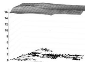
Figura 6.- Plano de presiones de Sector 35 después de los 55 cambios.
