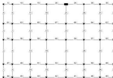
Figura 1.- Red Hipotética R28 con identificador de tubos.
