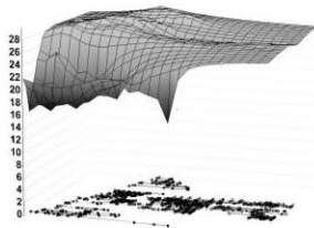
Figura 5.- Plano de presiones inicial de Sector 35.
