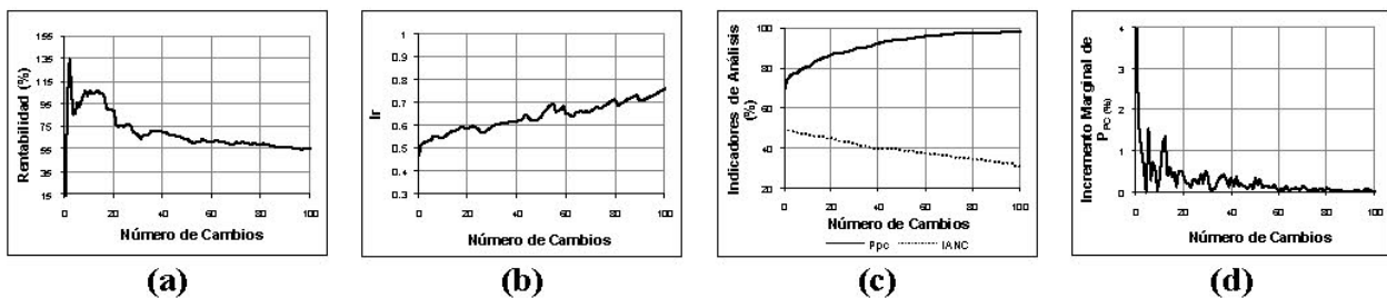
Figura 3.- Resultados red R28: (a) Rentabilidad, (b) I_r , (c) IANC y P_{PC} , (d) incremento marginal de P_{PC} vs. Número de cambios (para x_f = 0,5 ; período de amortización = 5 años)
